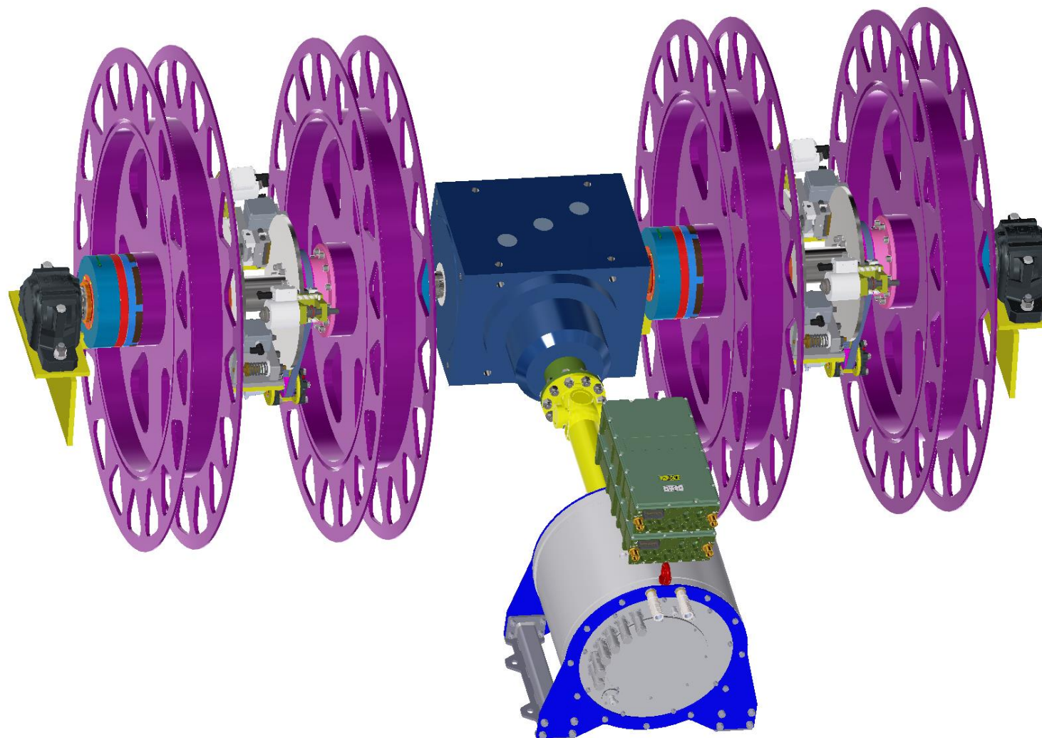
Rys. 2 Elektryczny układ napędowy bębnow linowych wyciągarki szybowcowej
